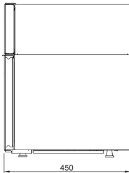
Rechterzij aanzicht
