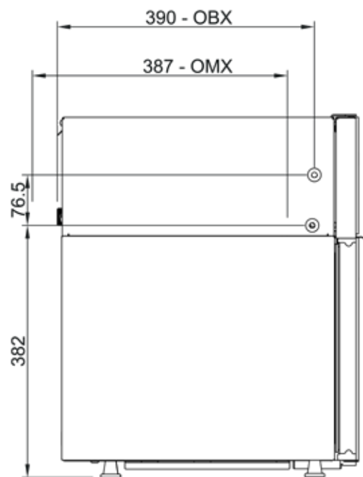
Linkerzij aanzicht
